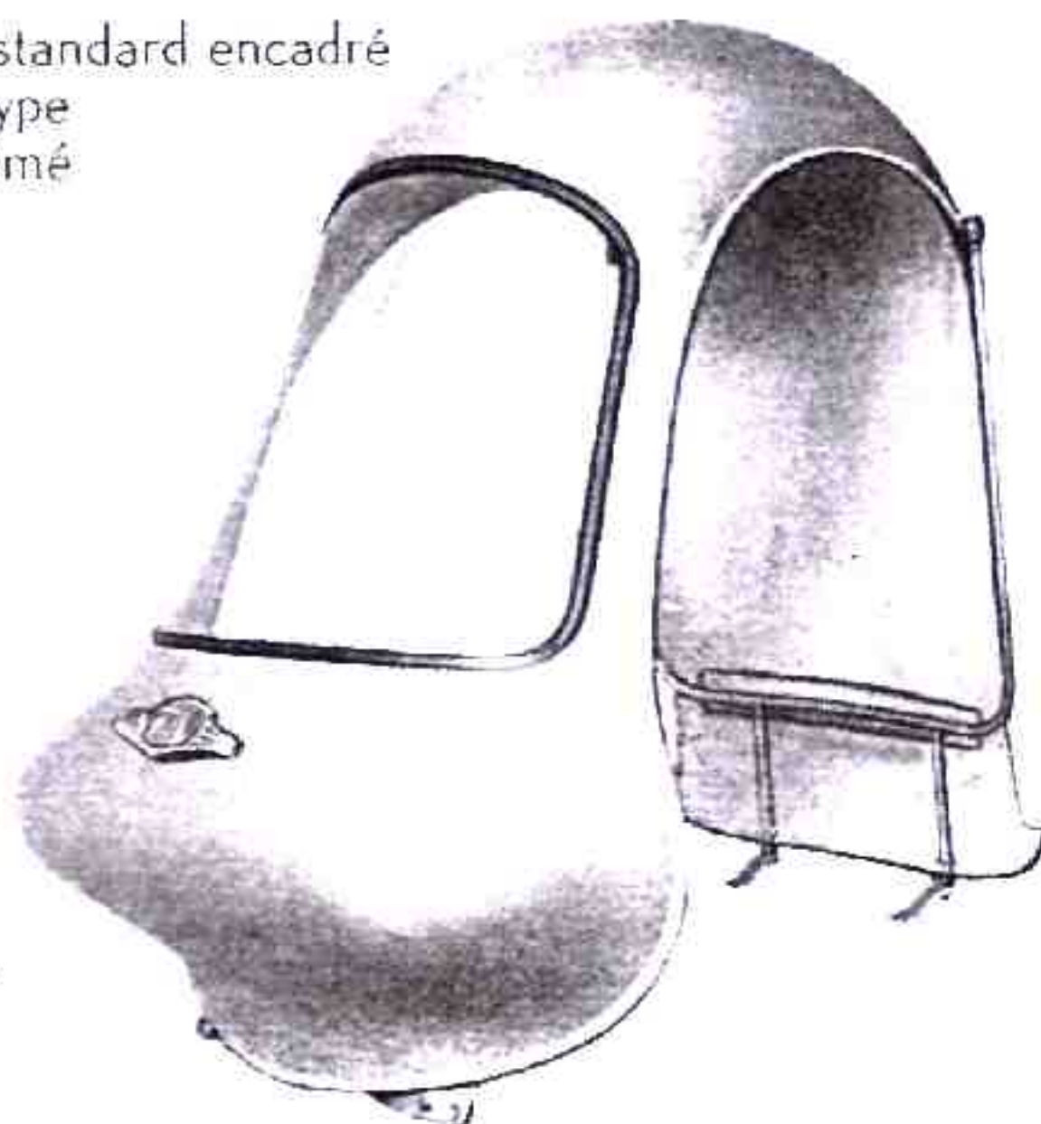
Réf. 10.265 - Capote métallique pour Tri, en peinture d'apprêt. Complète avec système de fixation et toile de protection arrière
