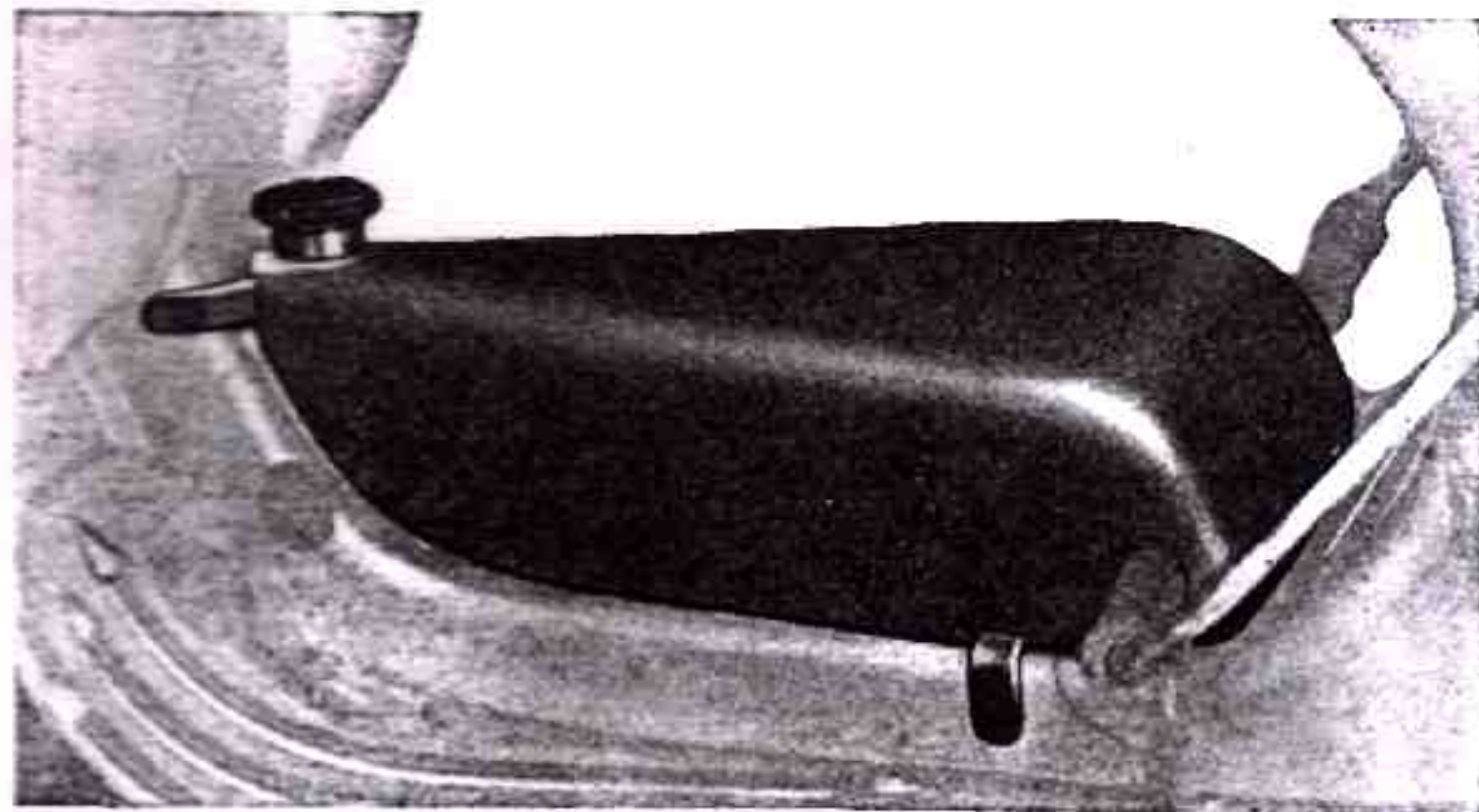
Réf. 10.106 - Bidon réservoir d'essence 6 litres, à poser sur plancher
