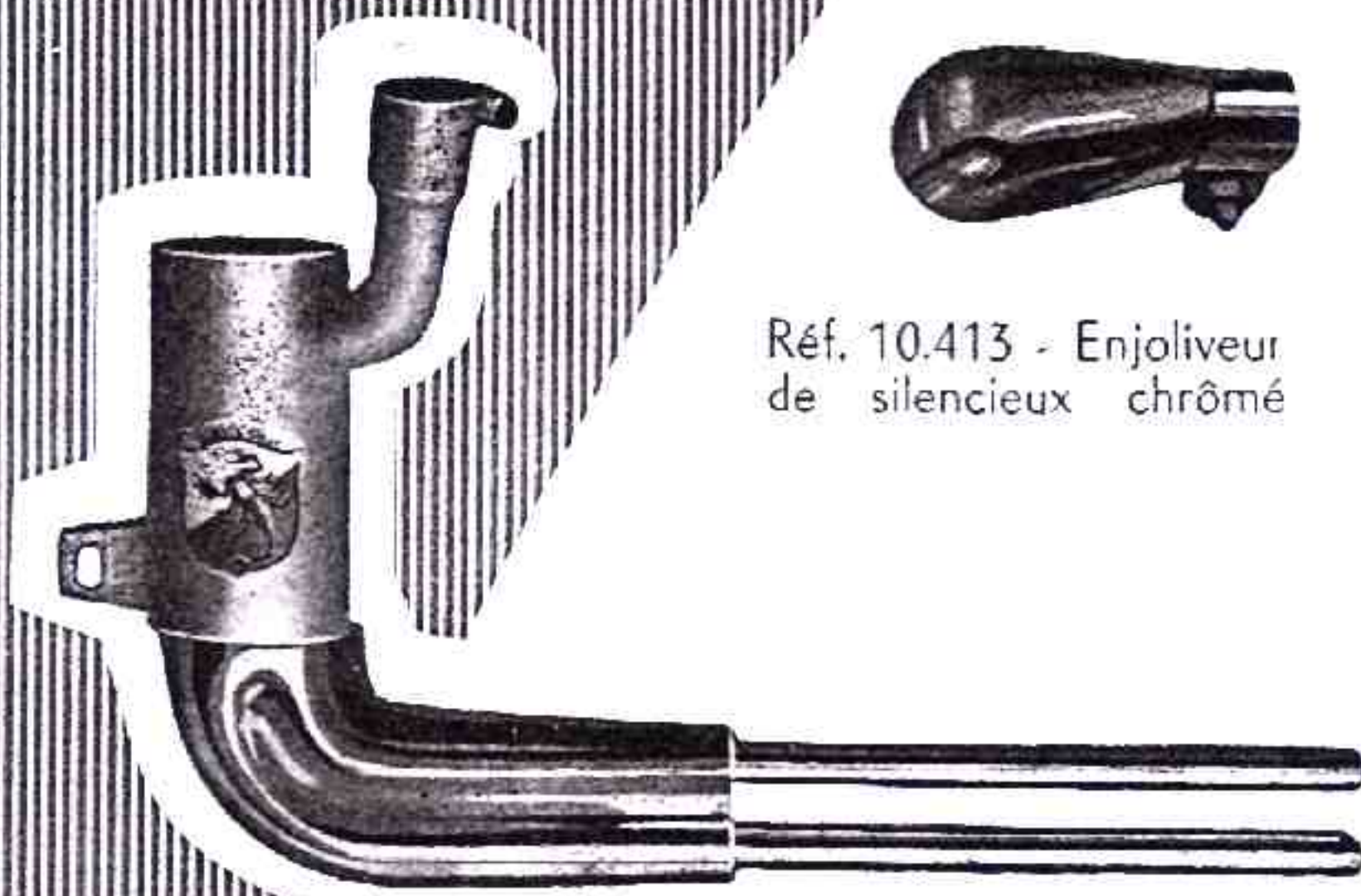
Réf. 11.914 - Tuyau d'échappement ABARTH chromé à double sortie pour modèle 54-55-56 Réf. 11.908 - Le même pour modèle 52-53
