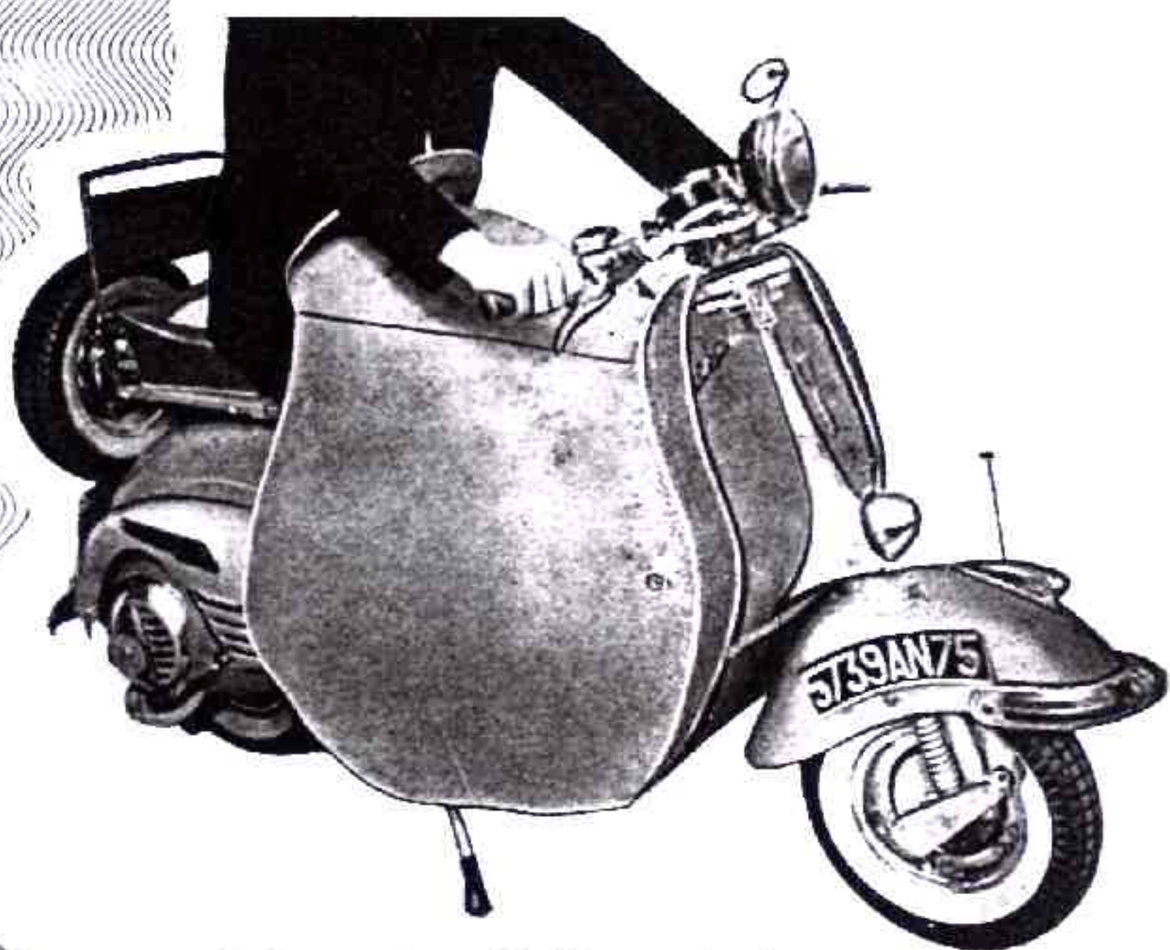
Réf. 11.906 - Tablier protecteur
