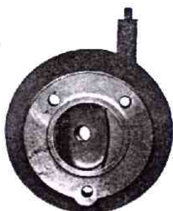
Réf. 10.264 Super-culasse VORTEX à haut rendement pour modèle 54
