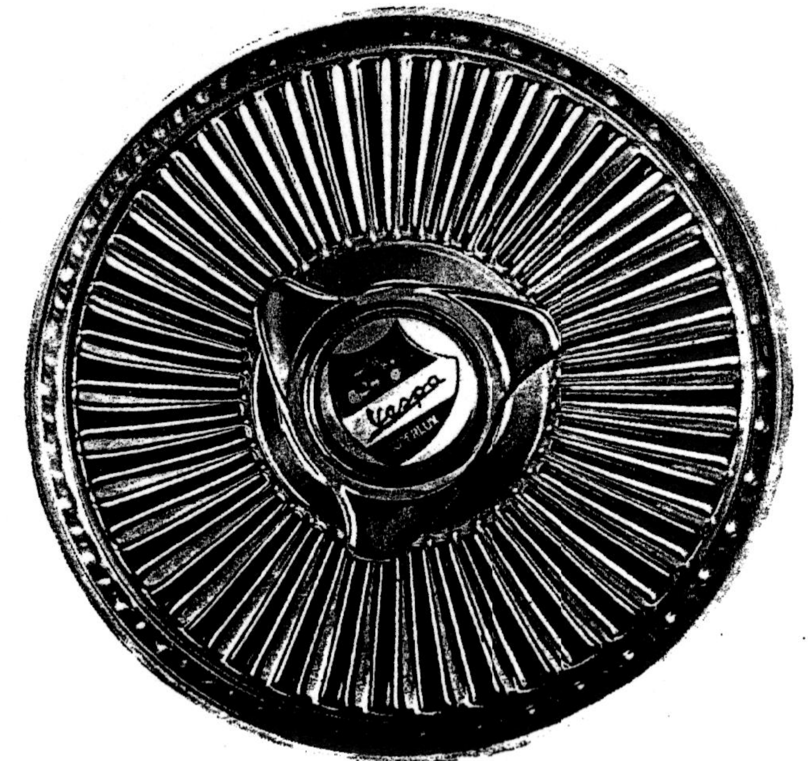
990 - Enjoliveur à Rayons, laiton chromé, avec Sous-Enjoliveur à Rayons Rouge.
